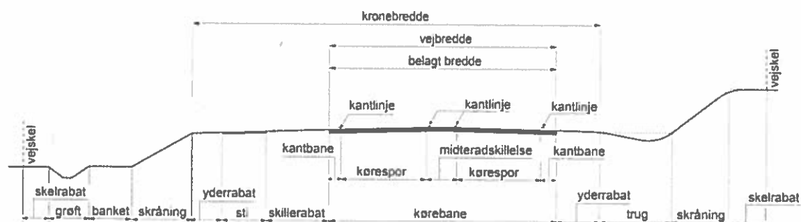
Figur 3.4 Tværprofilelementer for en vej uden midterrabat.
